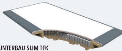
UNTERBAU SLIM TFK Höhe ca. 12 cm
